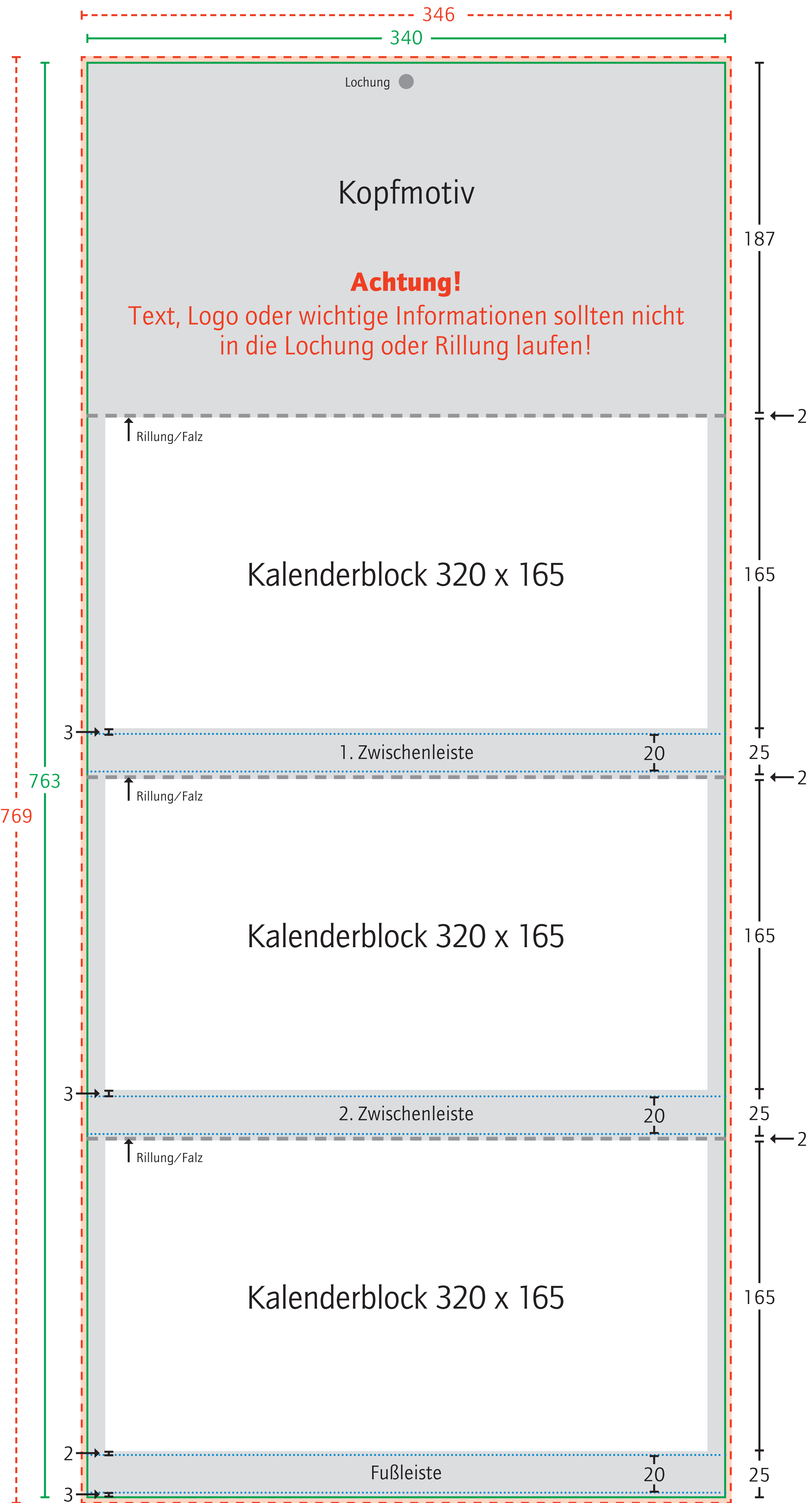
Alle Maße in mm
